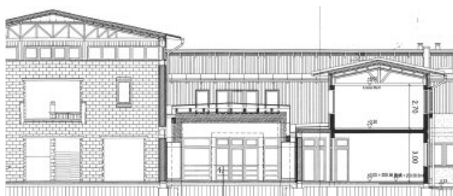
Iskolabővítés alaprajz és metszet. Tervező: Varga Tamás
